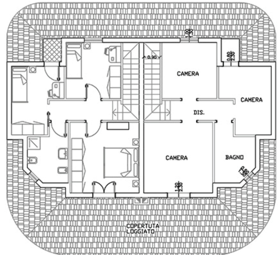
Primo Piano - Quadrivano
