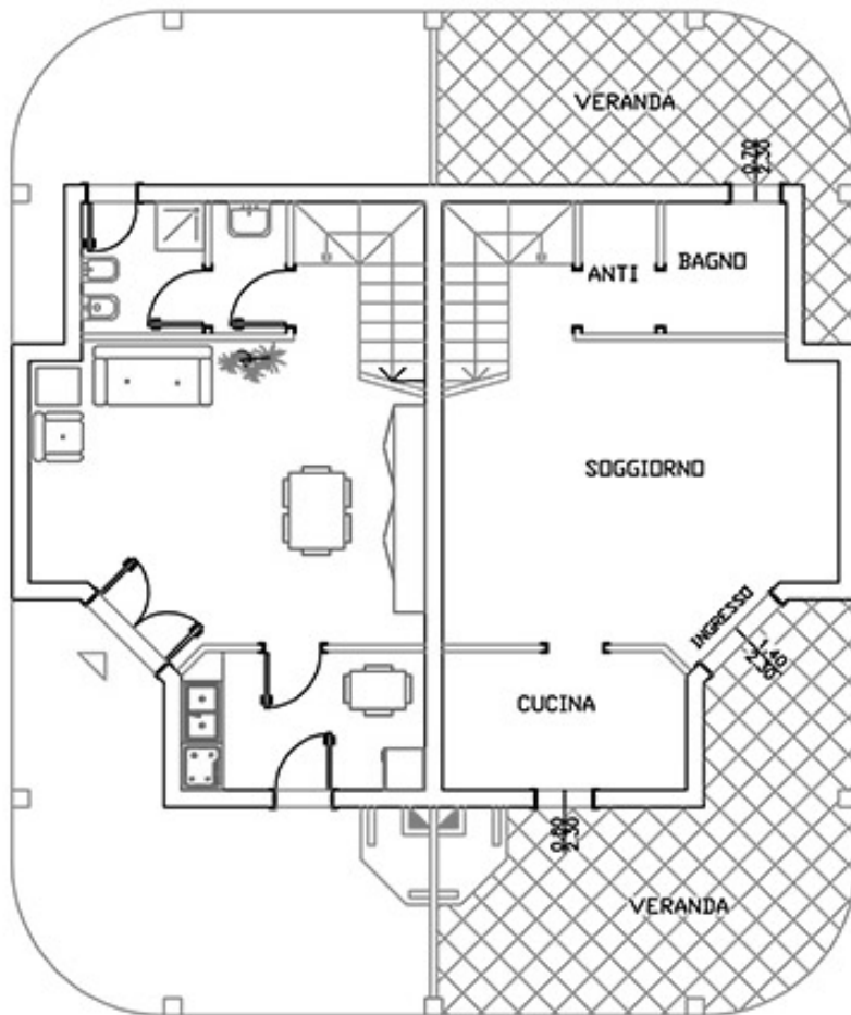
Piano terra - Trivano
