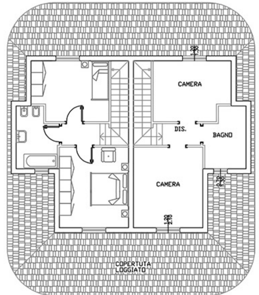
Primo piano - Trivano
